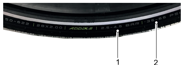
Abbildung 118: Fülldruck in bar (1) und psi (2)
