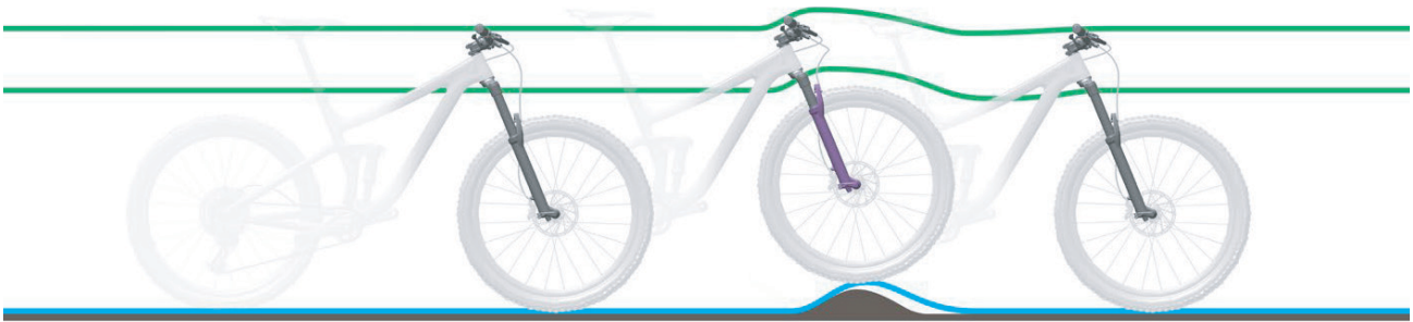
Abbildung 199: Zu harte Dämpfung der Federgabel bei Unebenheiten
