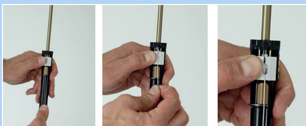
Abbildung 136: Seilzug aushängen
