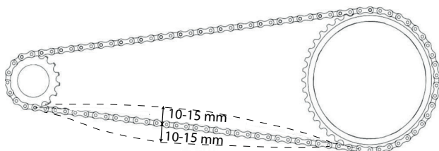
Abbildung 123: Kettenspannung prüfen
