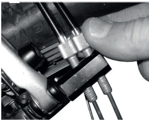
Abbildung 152: ROHLOFF-Naben Versionen mit interner Schaltansteuerung haben die Zugeinsteller am Zuggegenhalter
