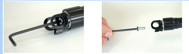
Abbildung 179: Ventilkappe herausdrehen
