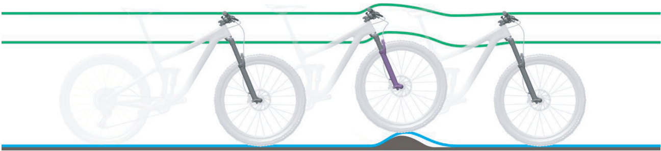
Abbildung 227: Zu harte Dämpfung der Federgabel bei Unebenheiten
