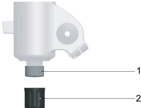
Abbildung 230: FOX Zugstufen-Schraube (1) unter Gabel-Kappe (2)
